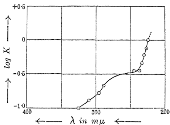
FIG. 4. \text{Na}\cdot\text{CH}_3\cdot\text{SO}_4 in water.
