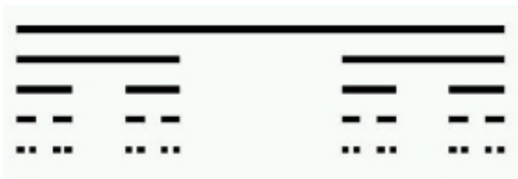
Figure A. Cantor set.
