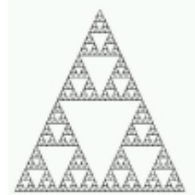
Figure B. Sierpinski gasket.
