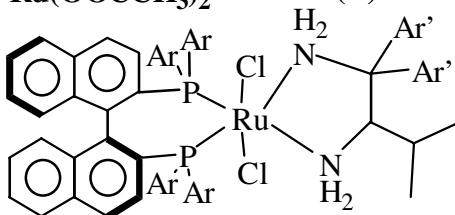
(R)-BINAP-RuX 2
