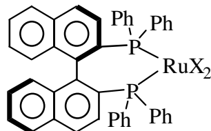
(R)-BINAP-RuX 2
