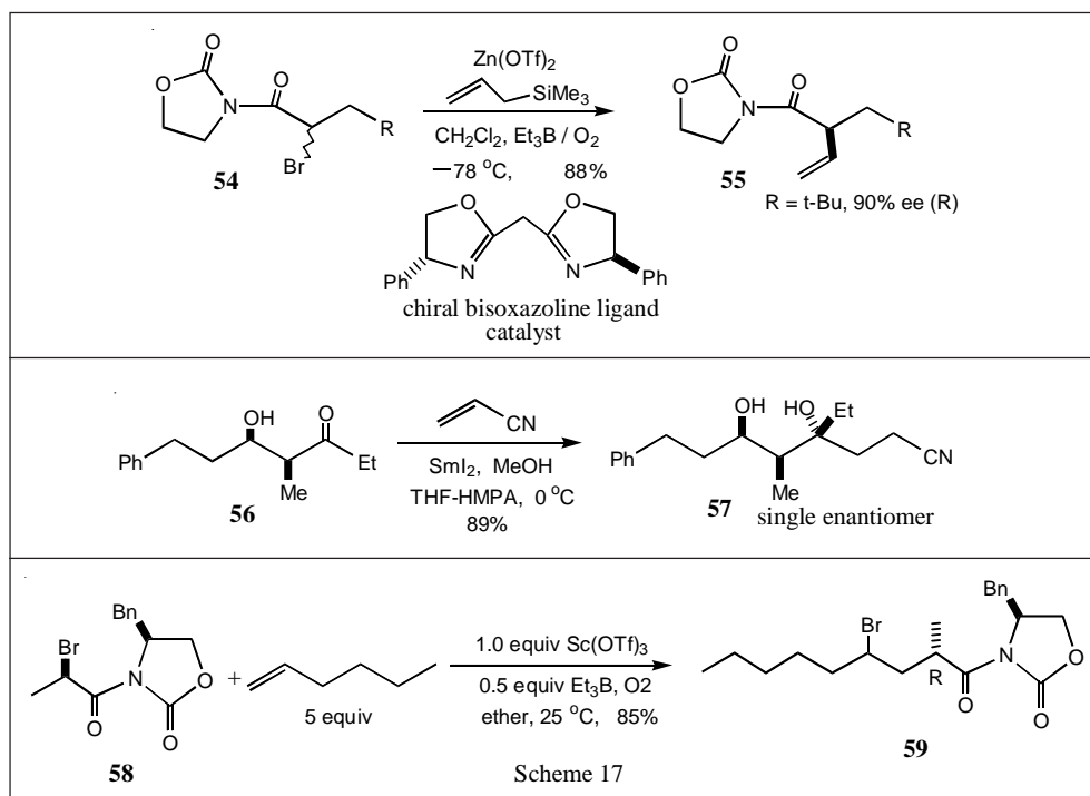
Schemes 15-17.
